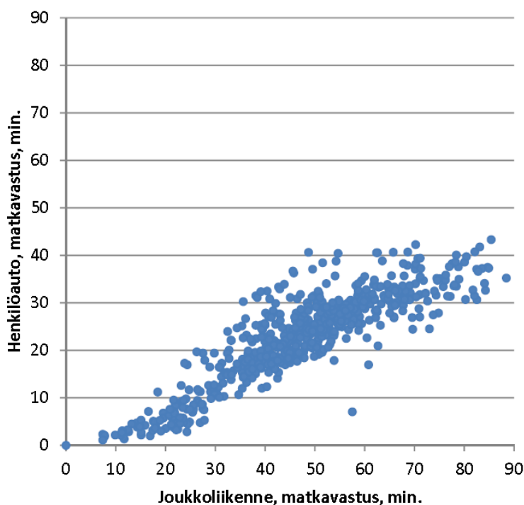
Kuva 10. Keskustasaavutettavuus Helsingin seudulla henkilöautolla ja joukkoliikenteellä (Laakso 2014, asiantuntijatyöpajan 28.11.2014 aineistoa).
