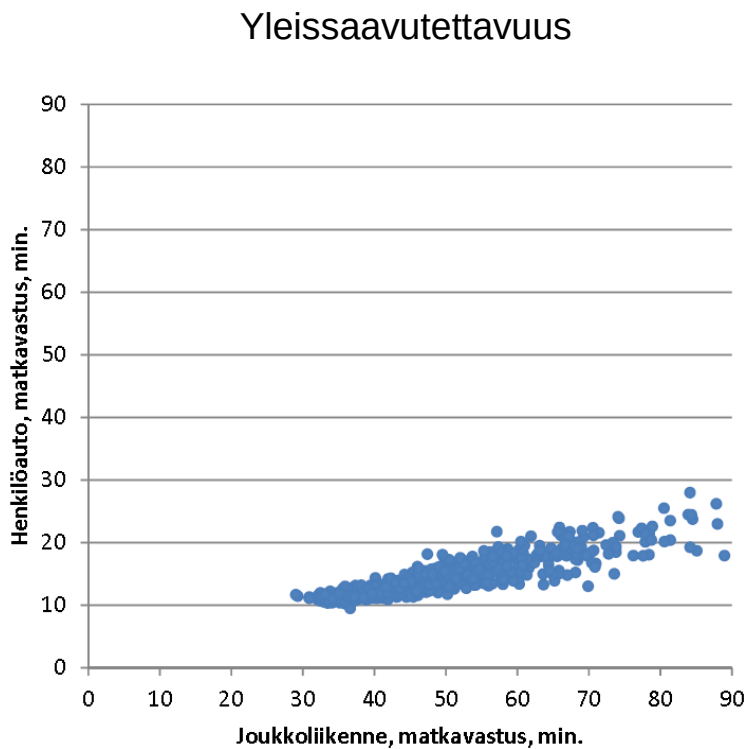
Kuva 11. Yleissaavutettavuus Helsingin seudulla henkilöautolla ja joukkoliikenteellä (Laakso 2014, asiantuntijatyöpajan 28.11.2014 aineistoa).
