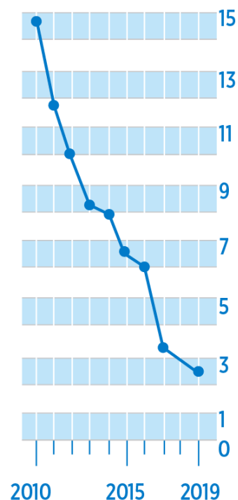
PM, pienhiukkaset
