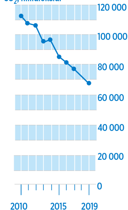
CO 2 , hiilidioksidi
