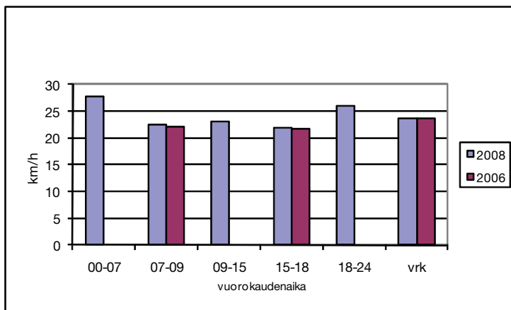
Kuva 3. Bussien keskimääräiset matkanopeudet arkena syksyllä 2008 ja 2006.
