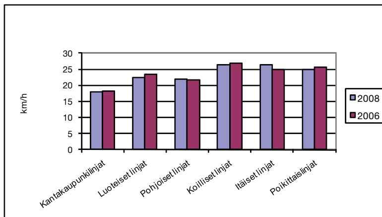
Kuva 4. Bussiliikenteen keskimääräiset matkanopeudet linjastoosittain arkena syksyllä 2008 ja 2006.
