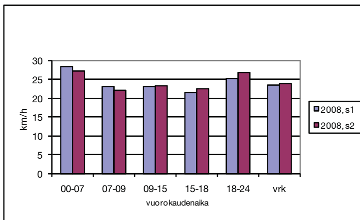
Kuva 1. Bussien keskimääräiset matkanopeudet ajosuunnittain arkena syksyllä 2008.
